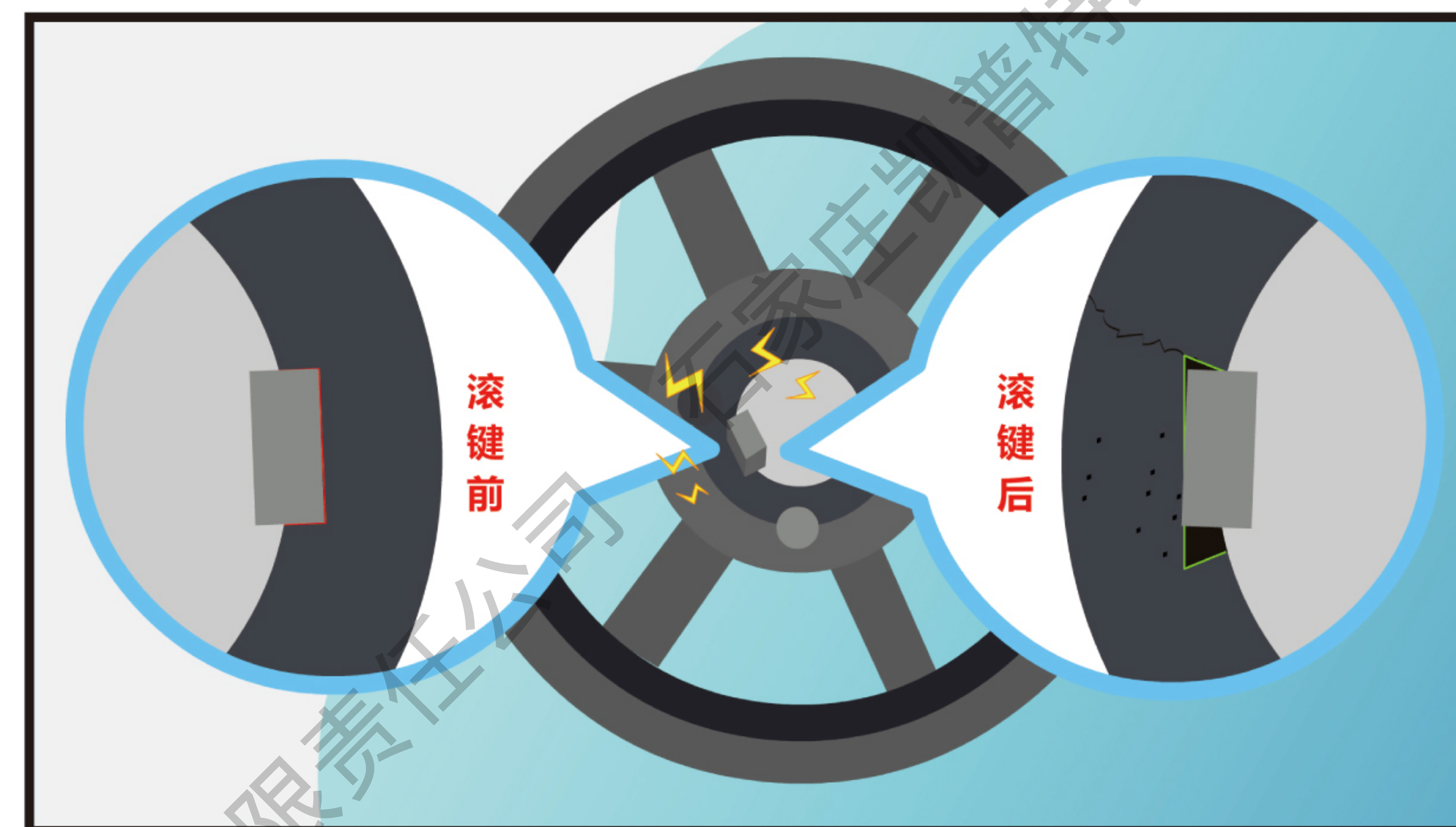
⑩铸铁材质锥套键槽容易发生“滚键”
