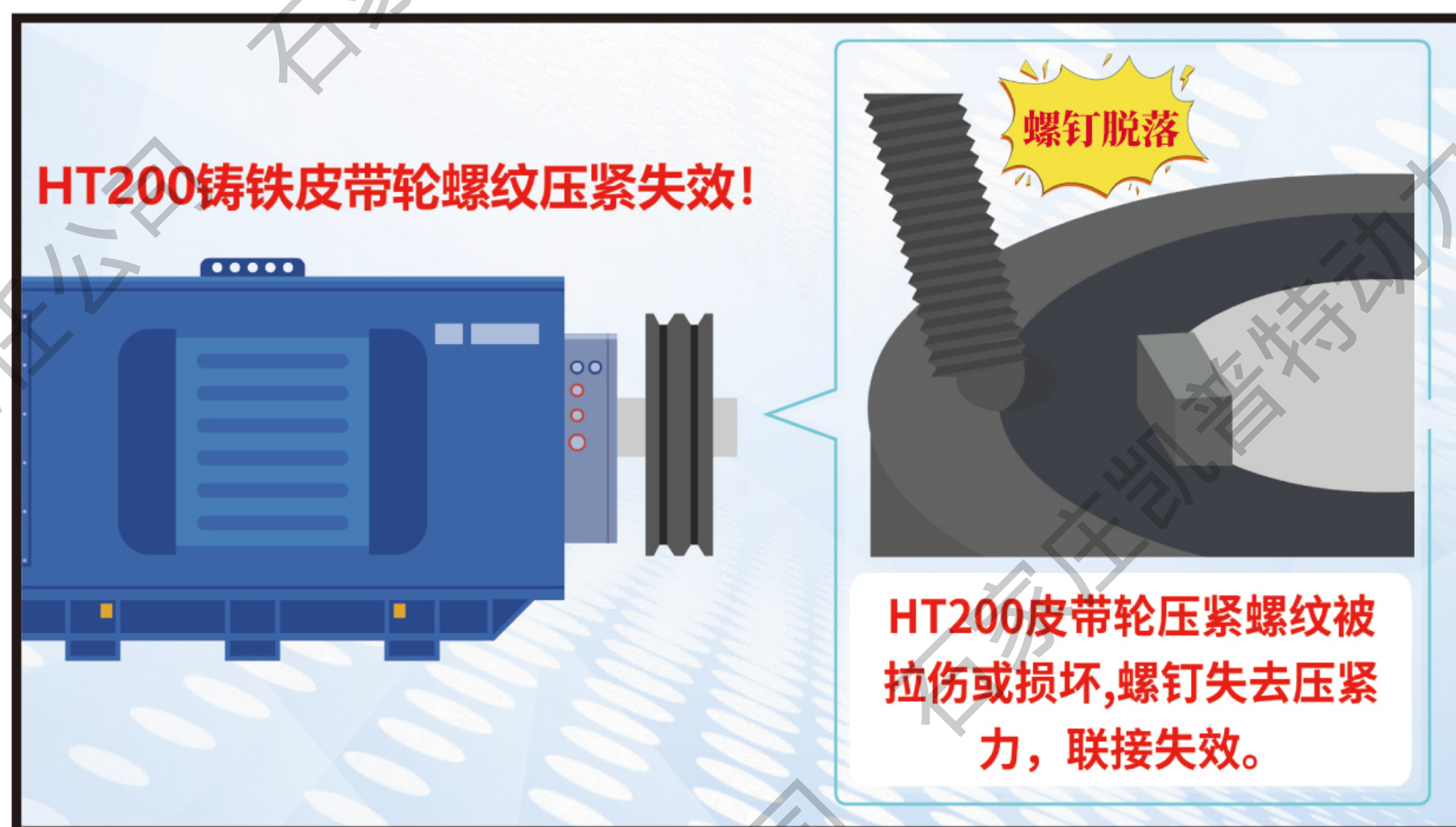
⑮螺孔“滑扣”造成压紧螺纹失效而分离脱出
