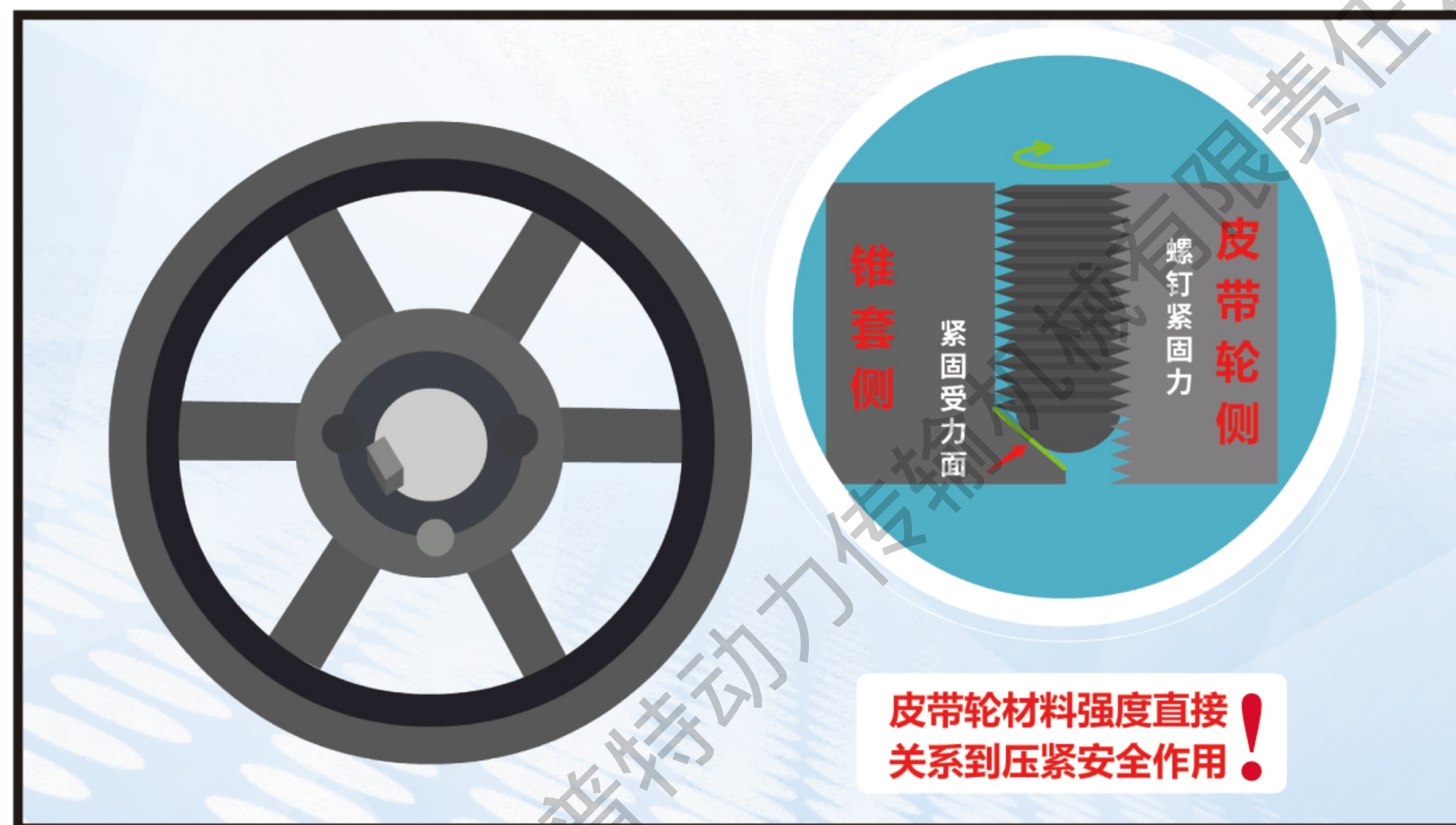
⑬锥套和皮带轮固定仅靠半边螺纹压紧
